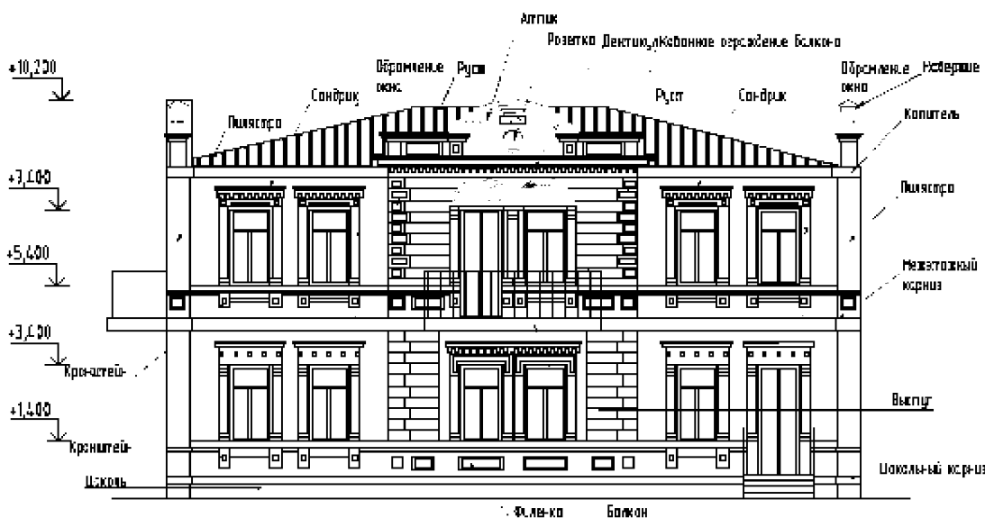
Схема. Проект предмета охраны «Особняк Тиц». Южный фасад по ул. Университетской.
